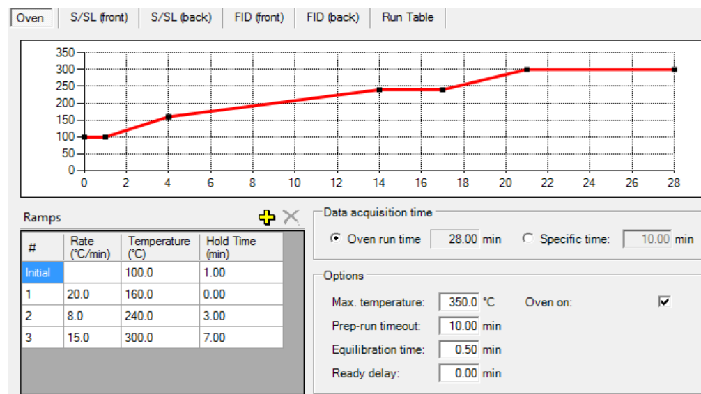
სურ.5 ქრომატოგრაფის სამუშაო რეჟიმი
